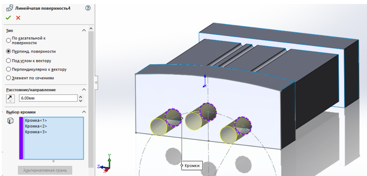
Рис. 19. Построение вытянутой поверхности
