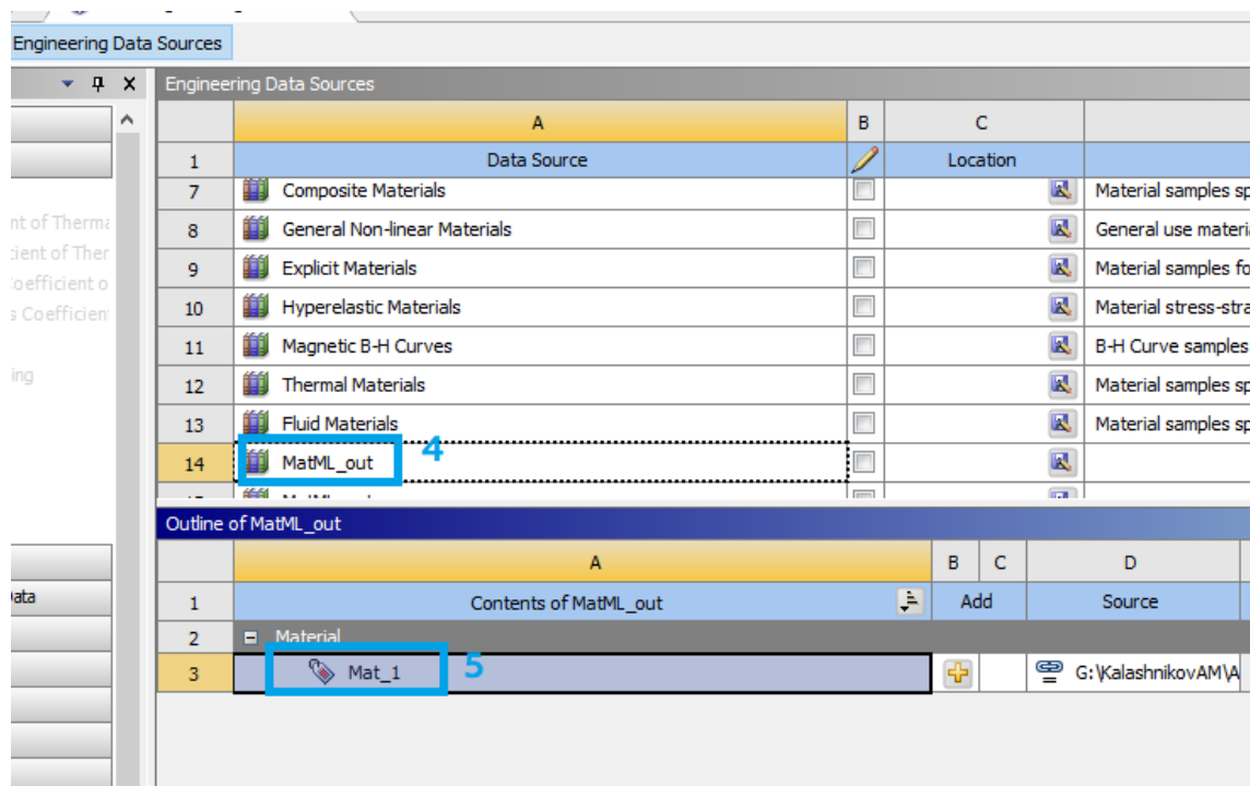
Рис. 14. Создание и добавление библиотеки материала
