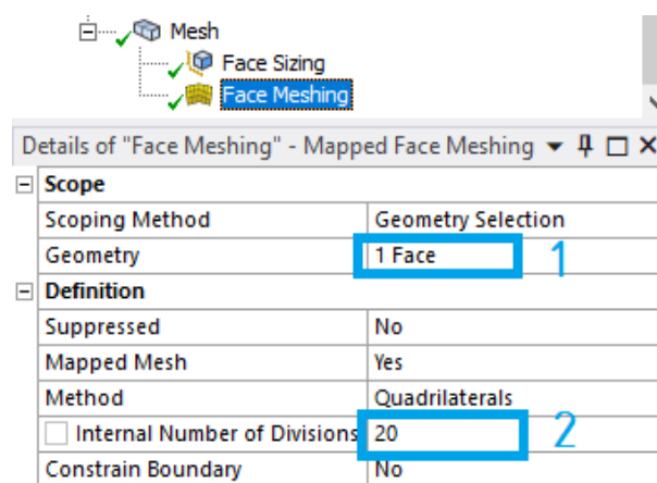
Рис. 10. Задание настроек сетки для участка № 1
