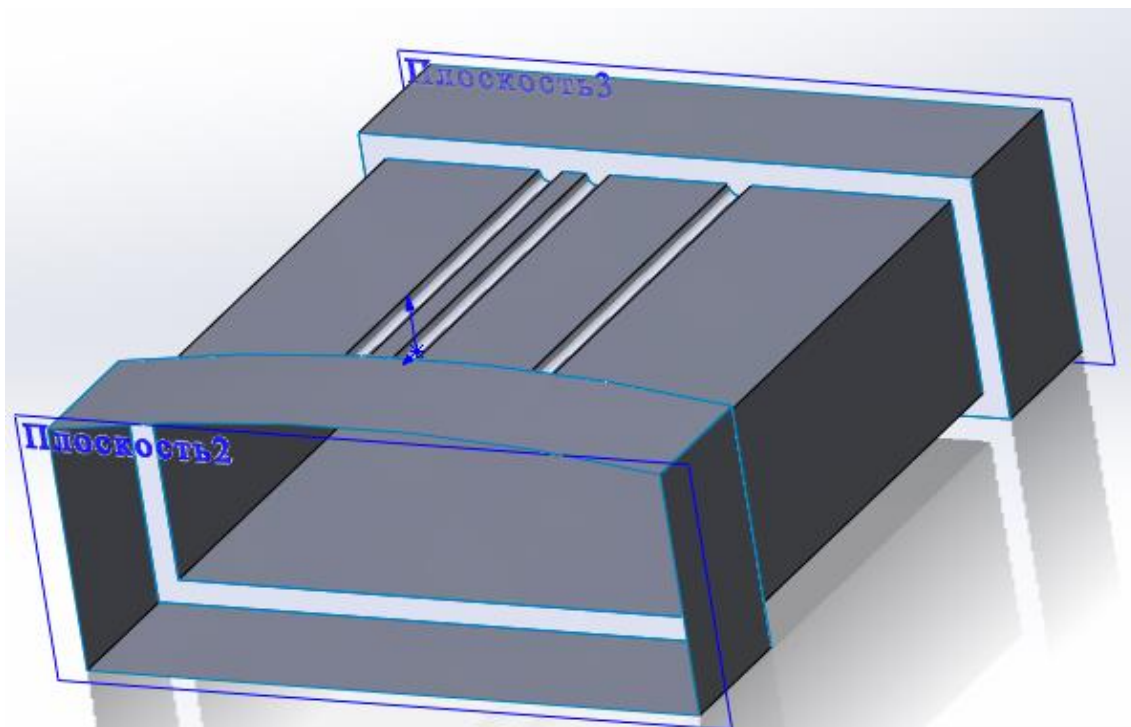
Рис. 14. Создание плоскостей
