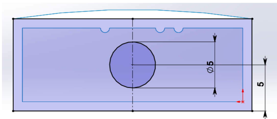
Рис. 15. Построение эскиза
