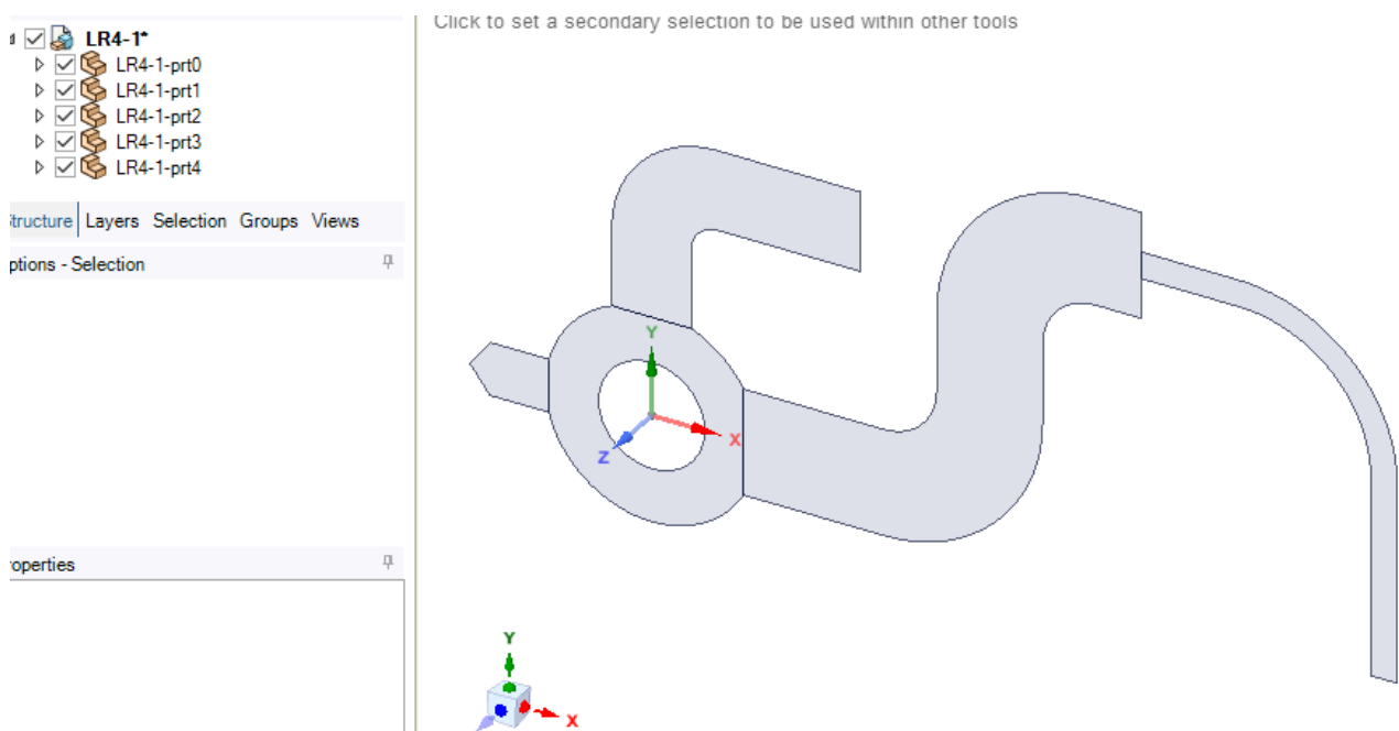
Рис. 8. Импорт геометрии
