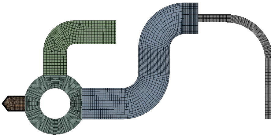
Рис. 16. Генерация сеточной модели
