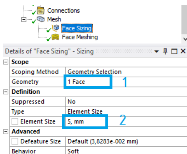
Рис. 10. Задание настроек сетки для участка № 1
