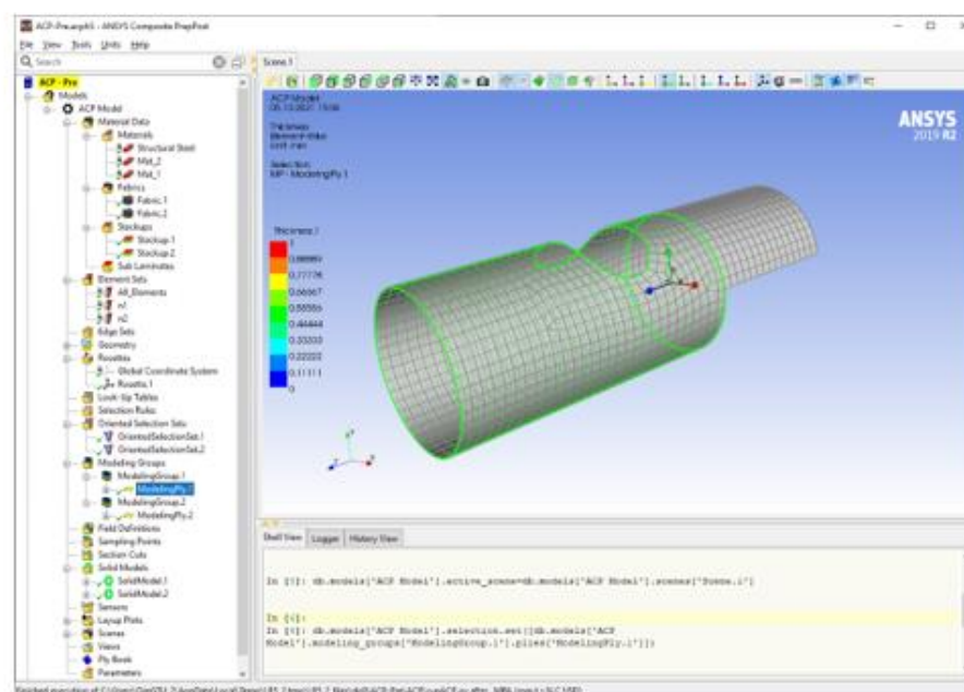
Рис. 7. Окно Setup
