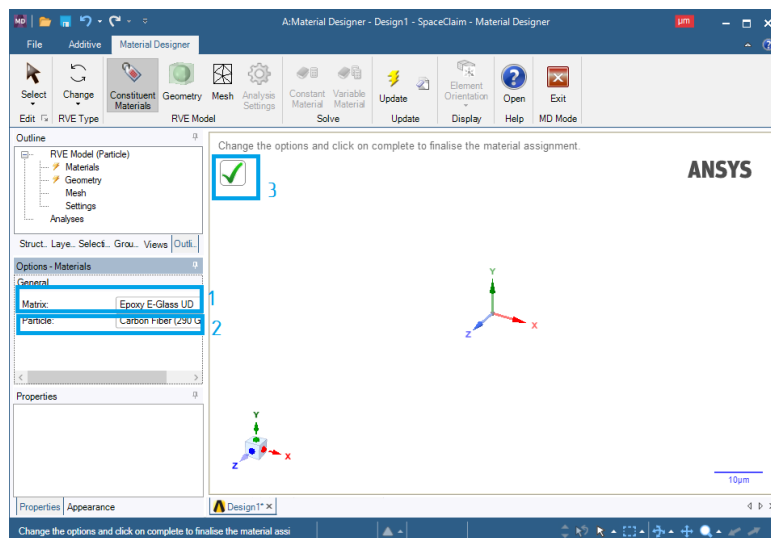
Рис. 8. Присвоение материалов
