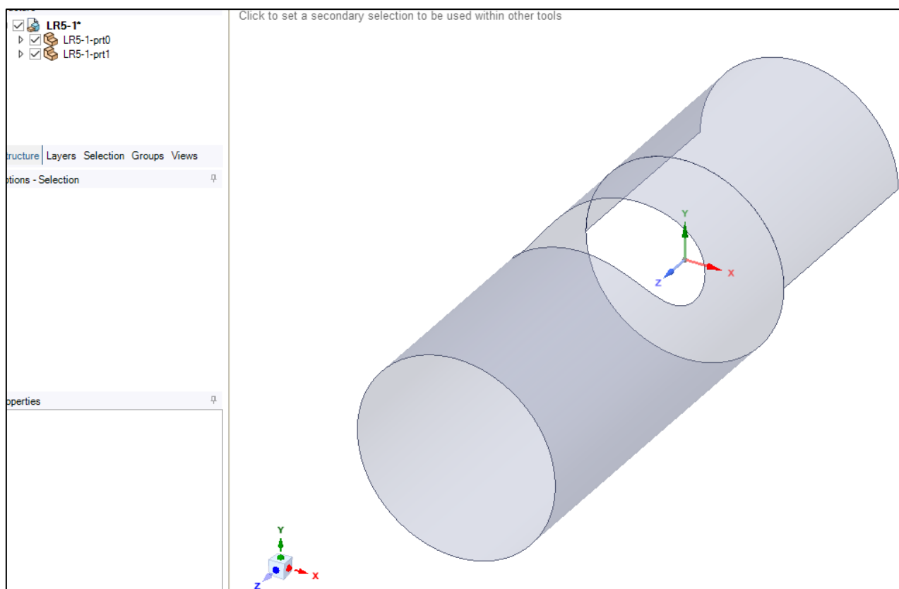
Рис. 16. Импорт геометрии
