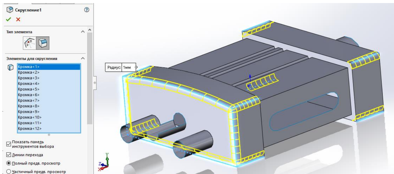
Рис. 28. Создание скруглений
