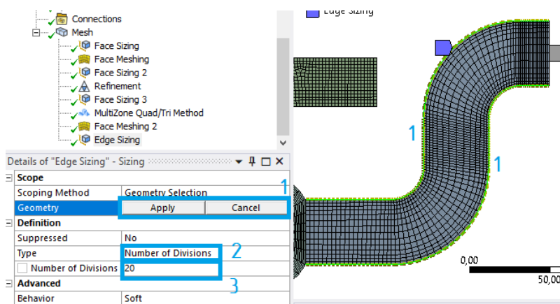
Рис. 14. Задание настроек сетки для участка № 4
